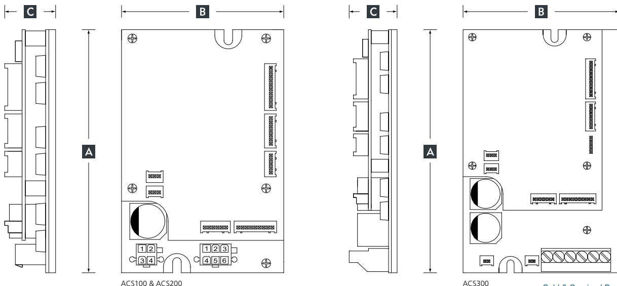
ACS100 & ACS200
