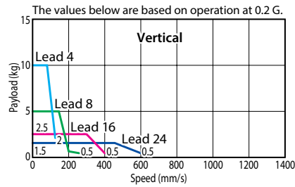
ERC3-RA6C
